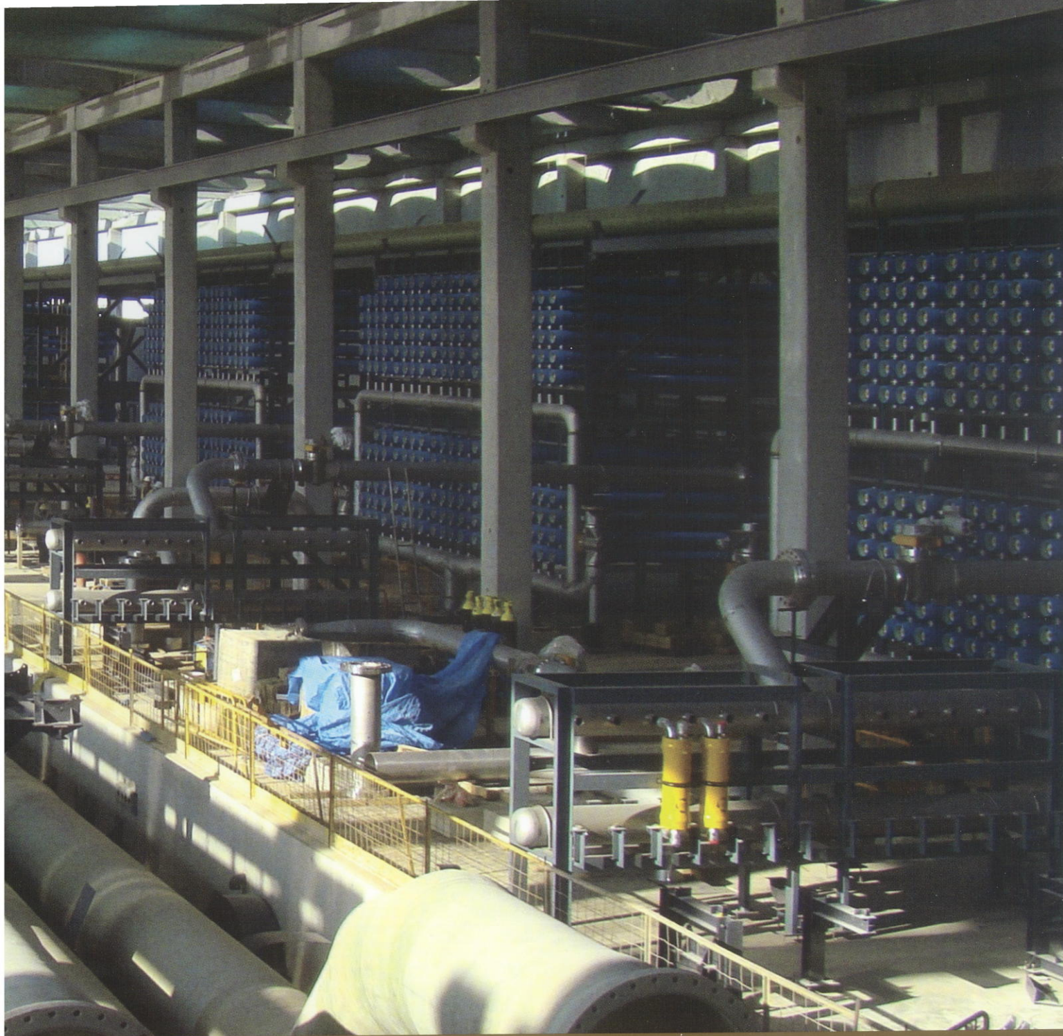
Edifici d'osmosi de la nova dessalinitzadora del Prat de Llobregat
