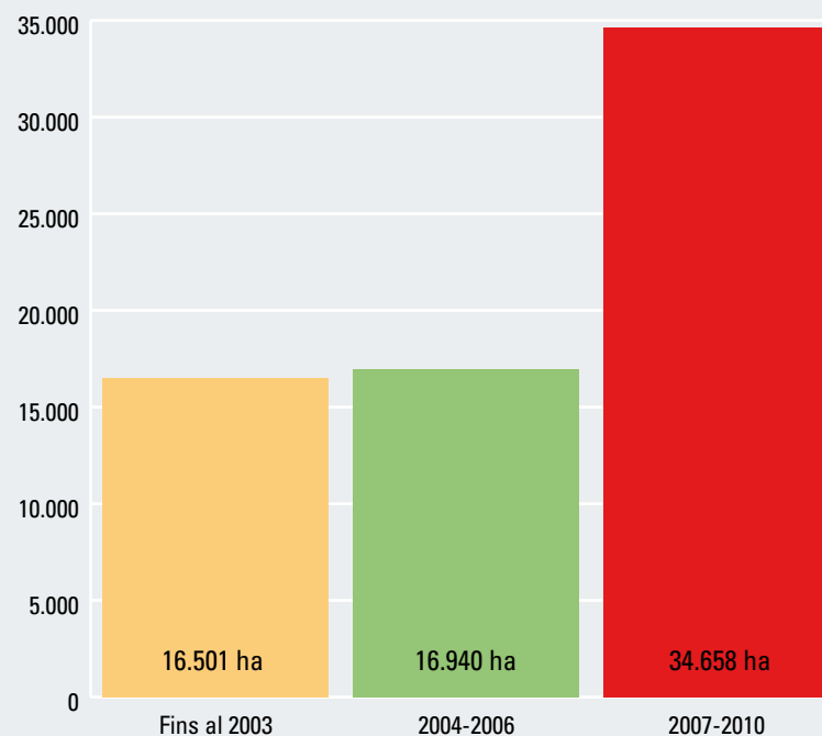
Gràfic 3. Regadius modernitzats posats en servei. 2003-2010 (ha). *2010 previsió
